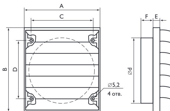
Размеры, мм
